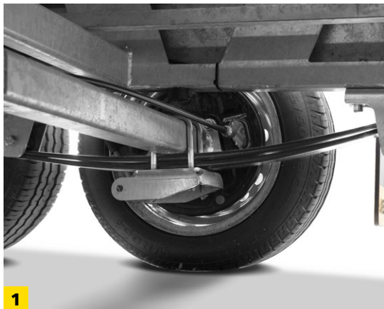
Parabelfeder
